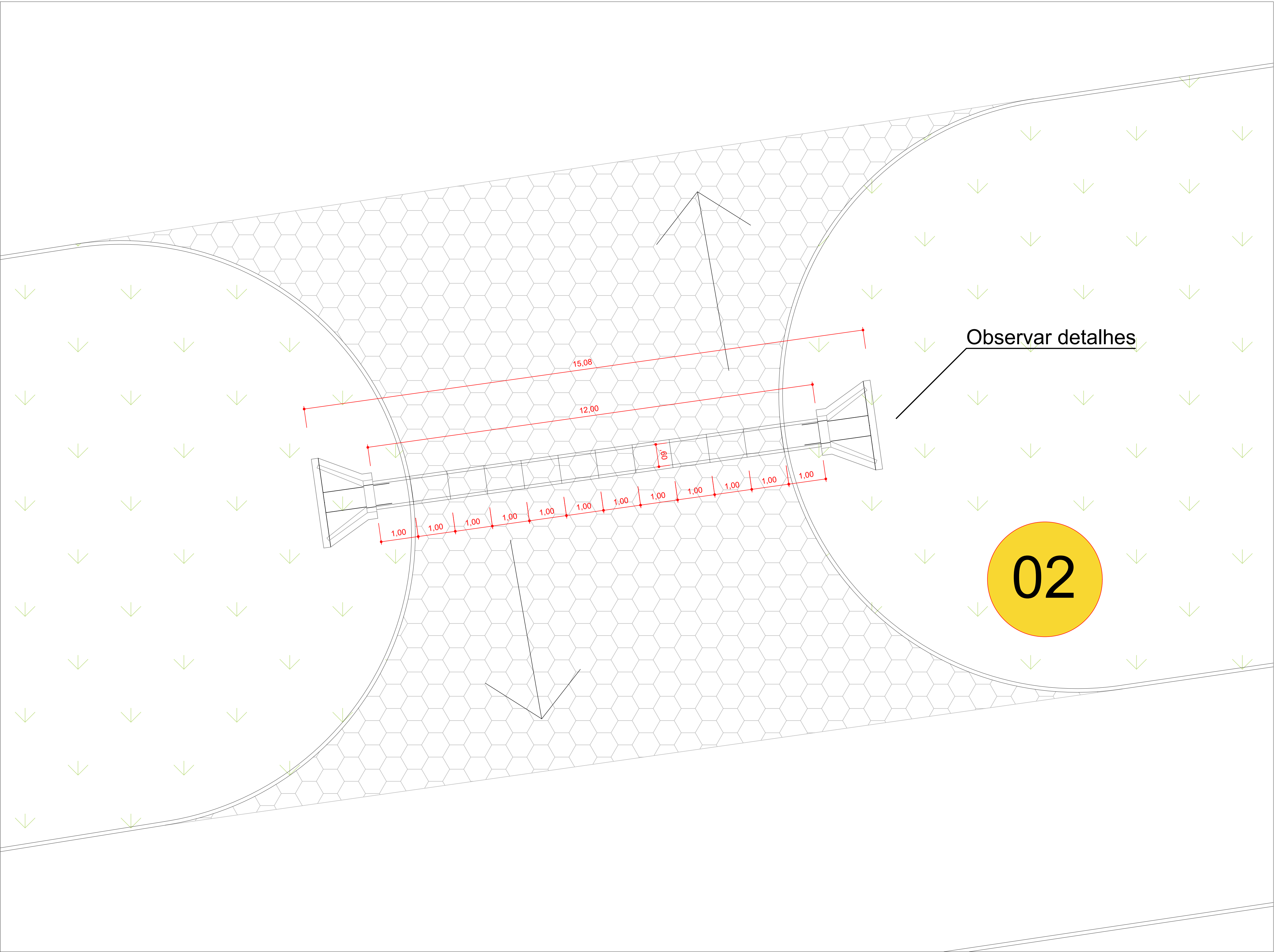
PLANTA BAIXA PLUVIAL RETORNO 03 ESC.: 1:75
